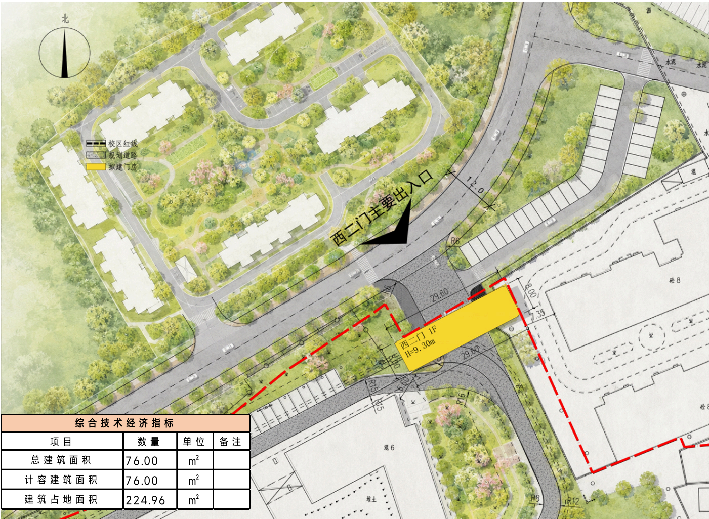
湖北师范大学西二门建设项目建筑设计方案规划设计平面图
