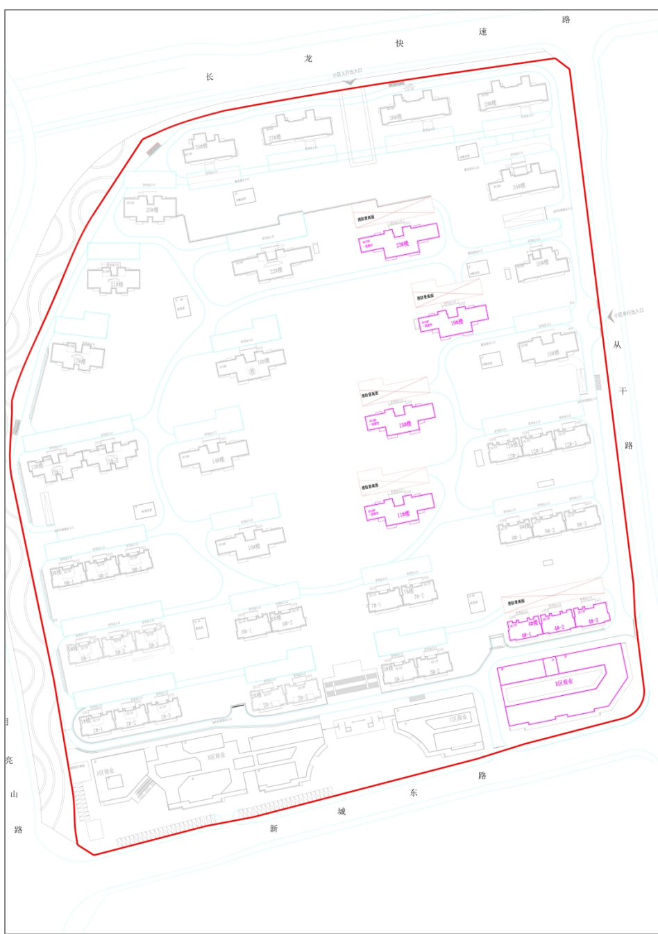
原规划审批总平面图
