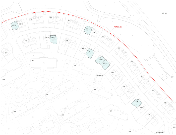
图 2：实测竣工总平面图
