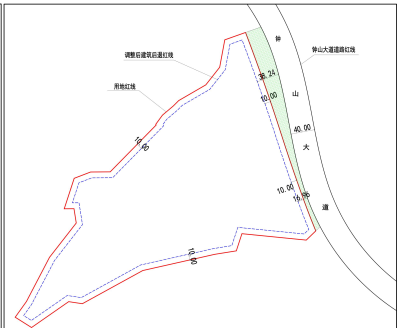
调整后建筑后退红线图：
