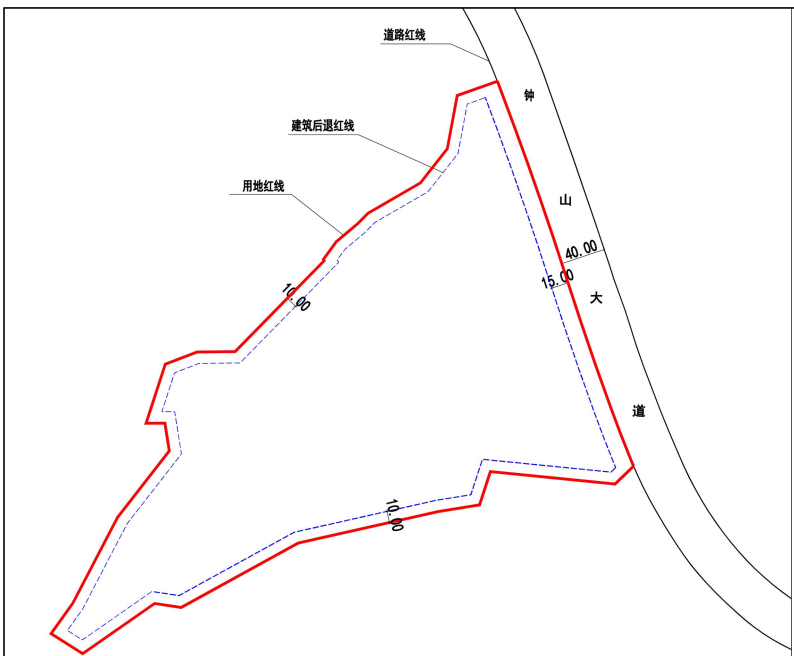
调整前建筑后退红线图：
