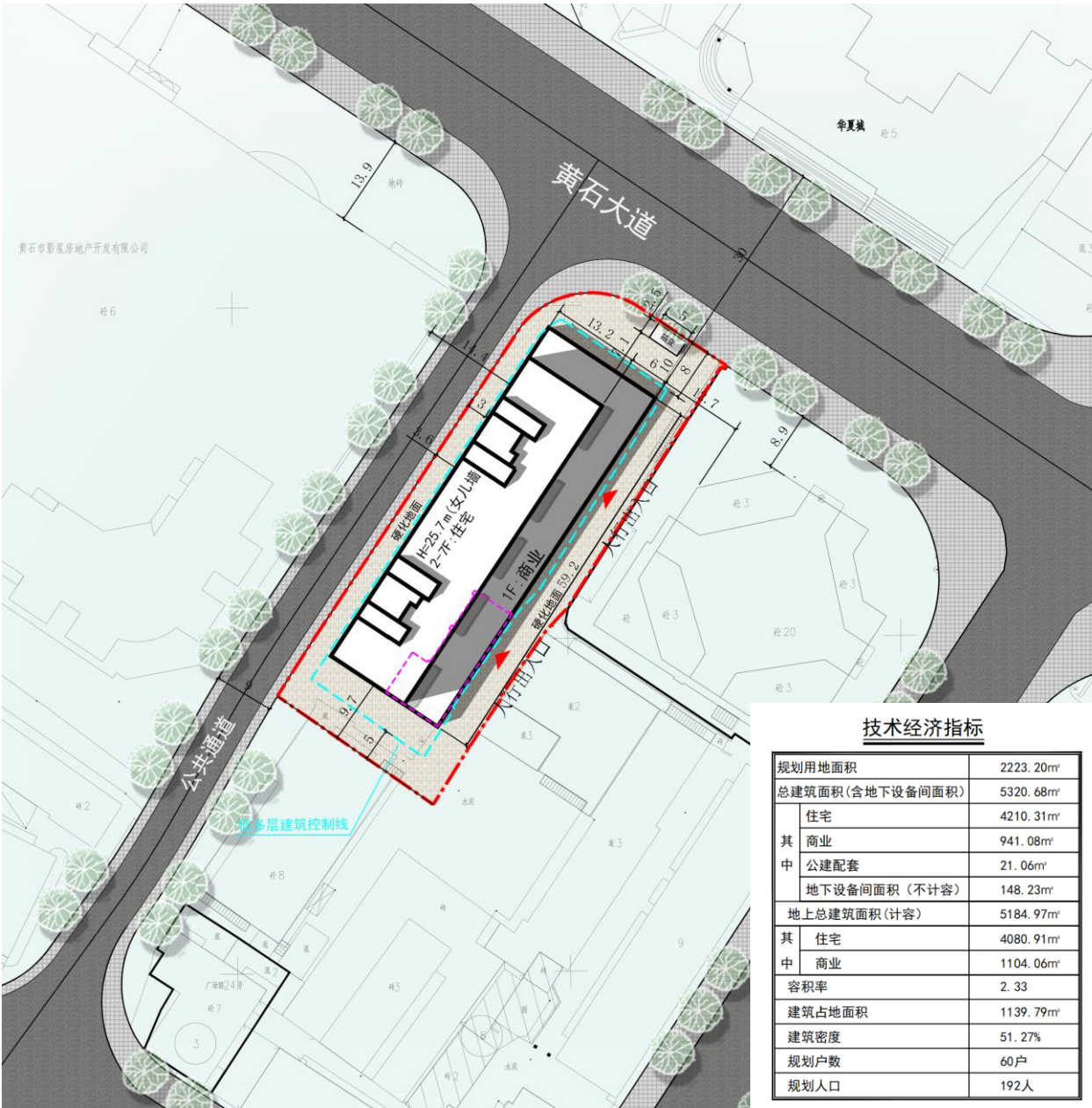
规划总平面
