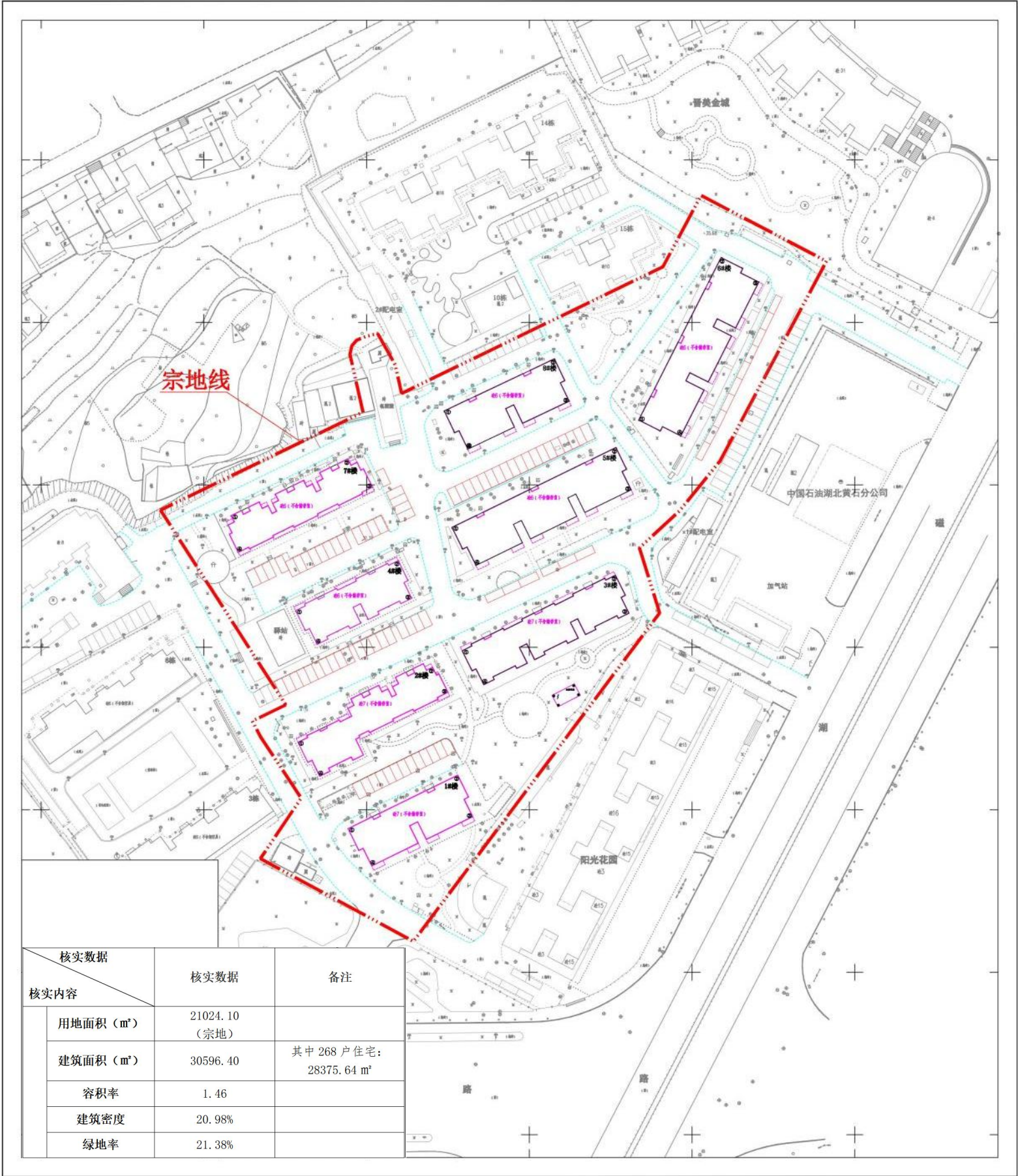
一、竣工总平面图
