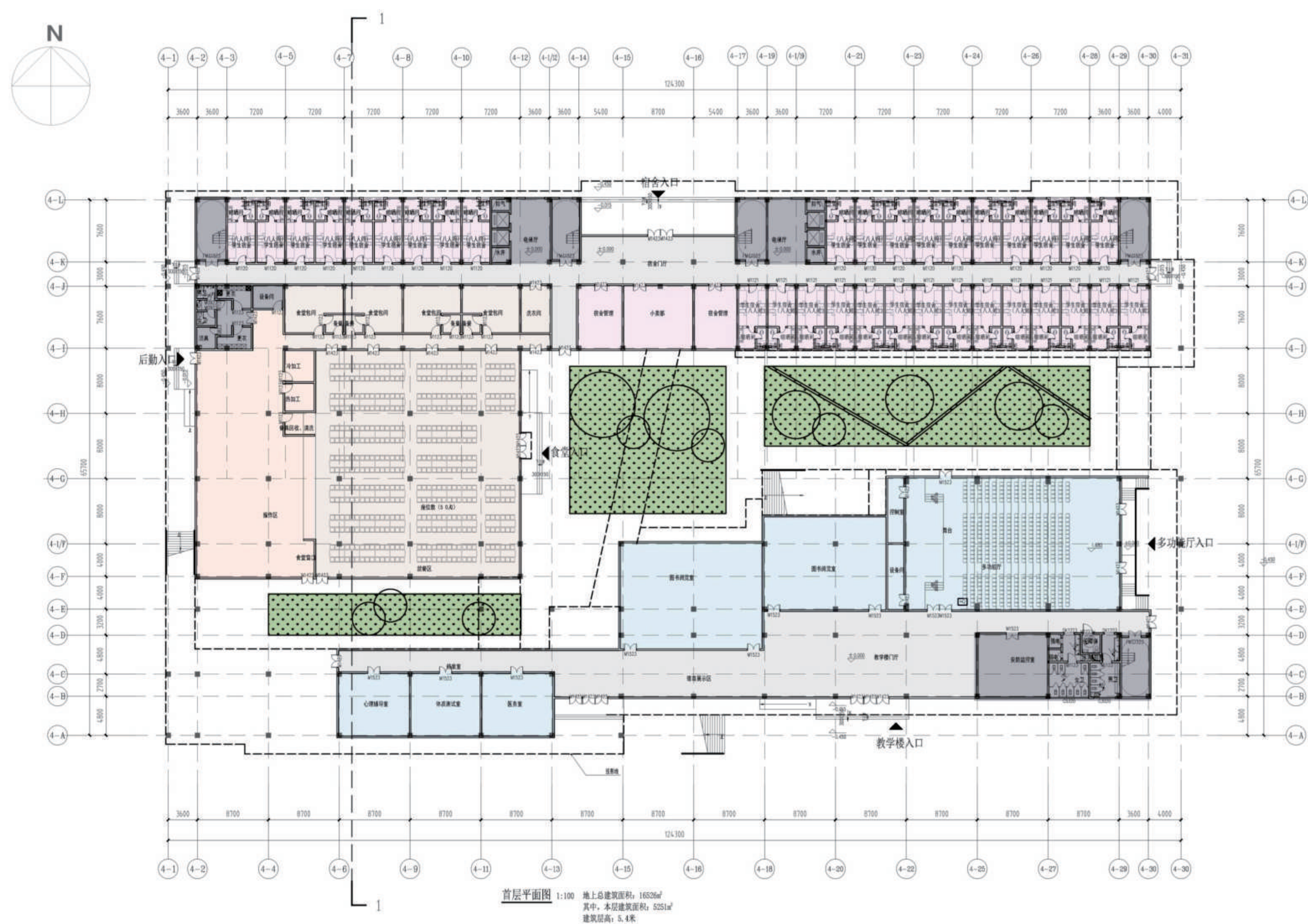
五、一层平面图
