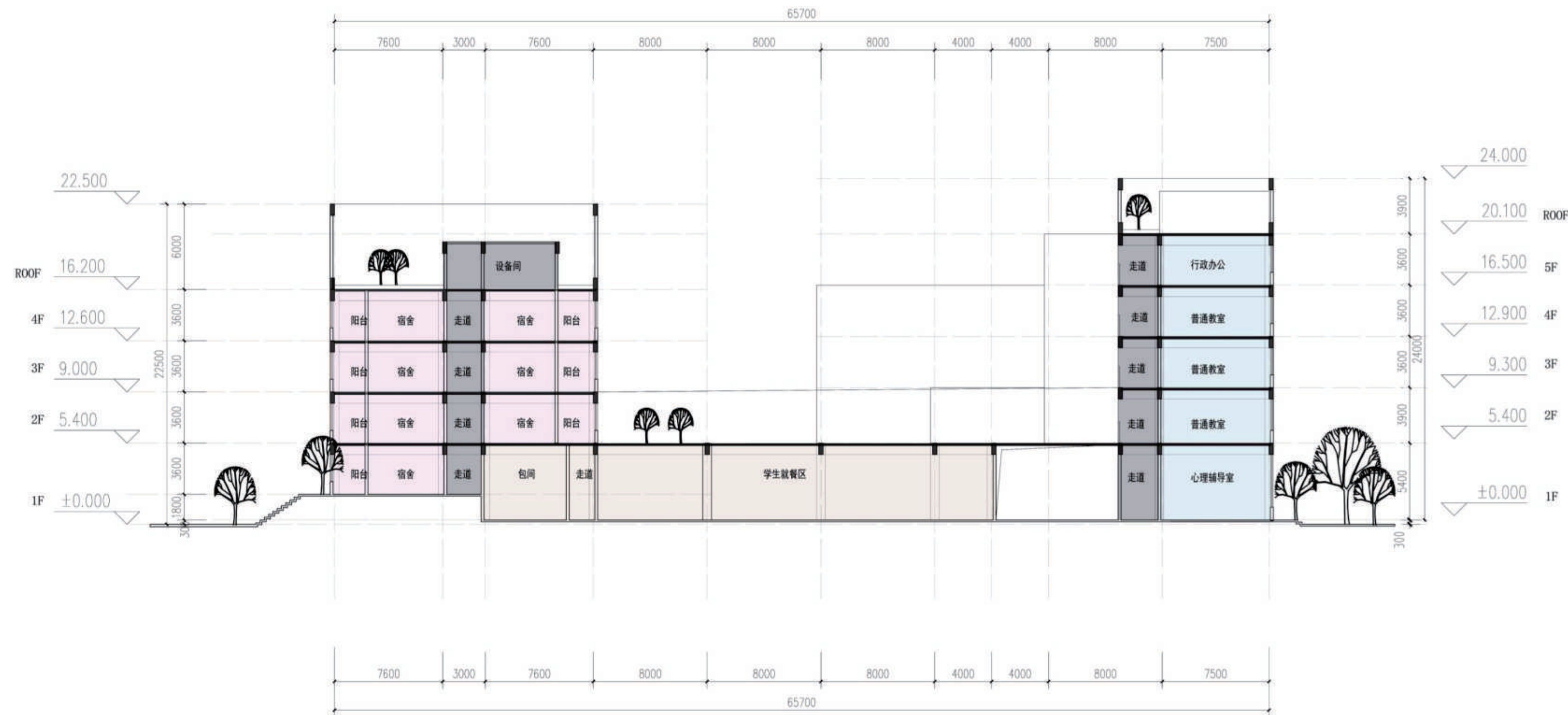
六、剖面平面图
