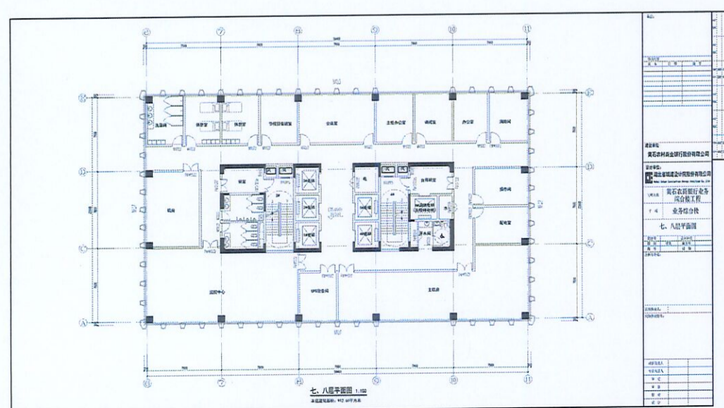
七、八层平面图
