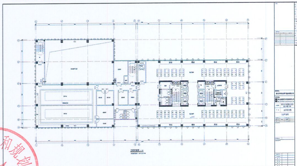
五、六层平面图
