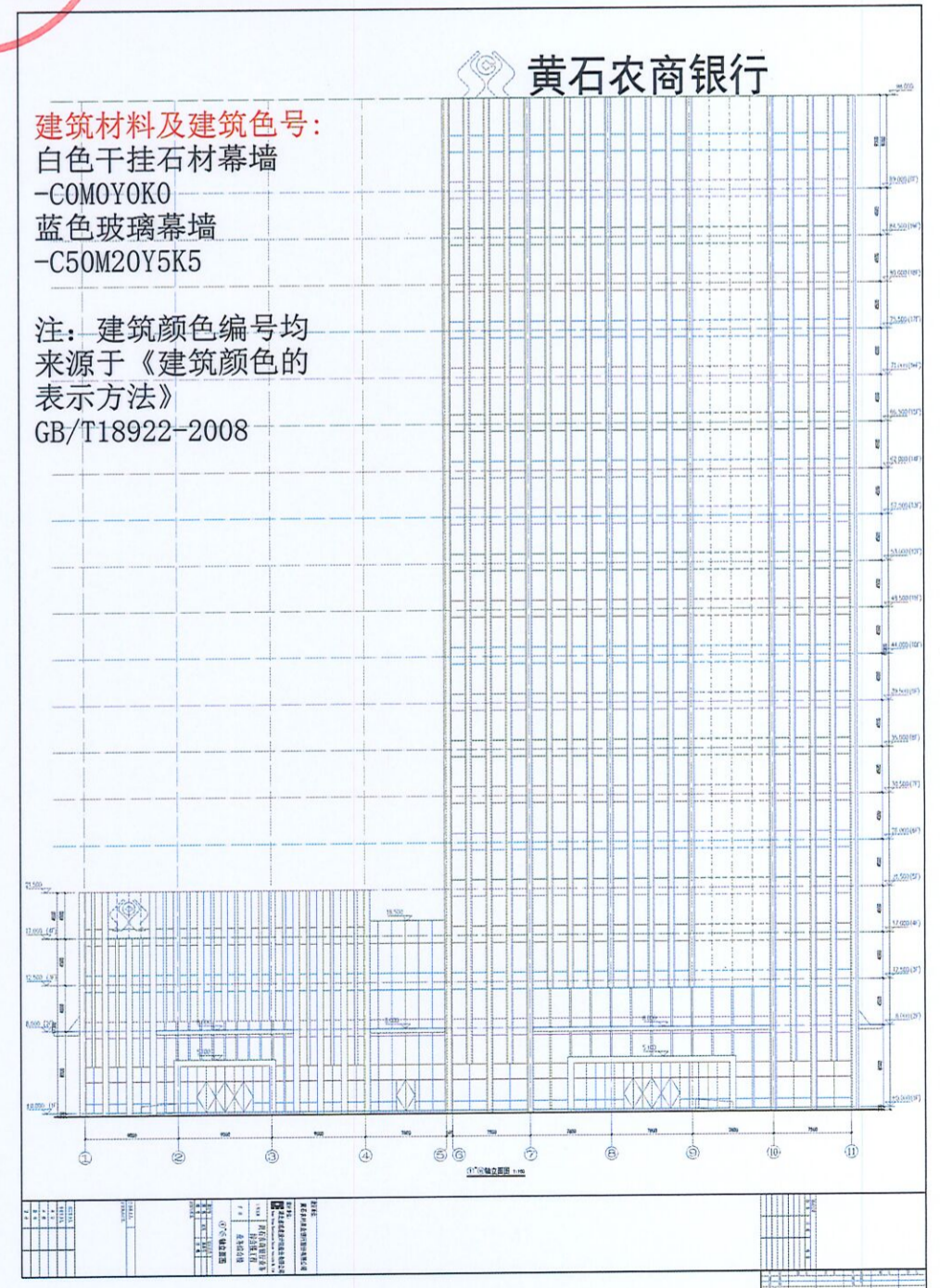
业务综合楼立面图
