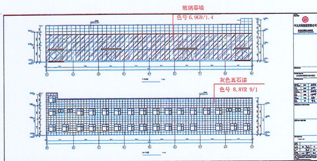
四. 综合多功能展厅立面图
