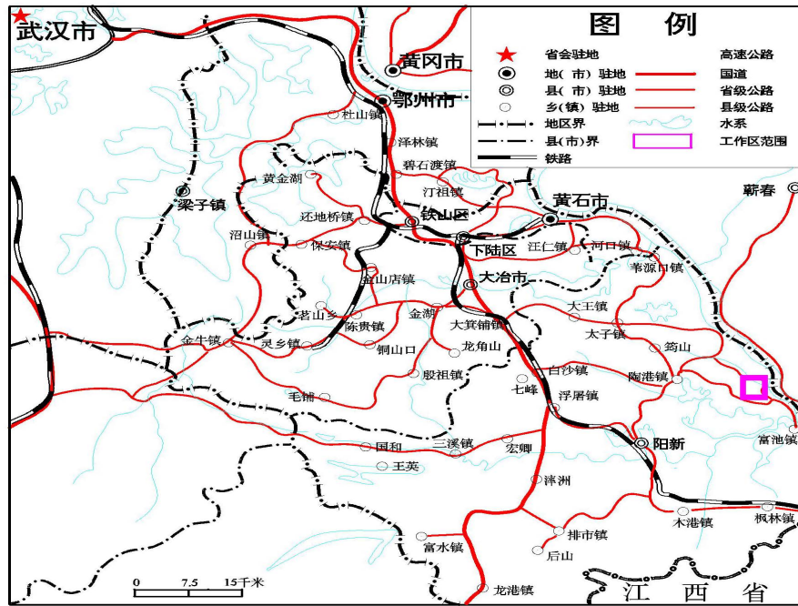
矿区交通位置图
