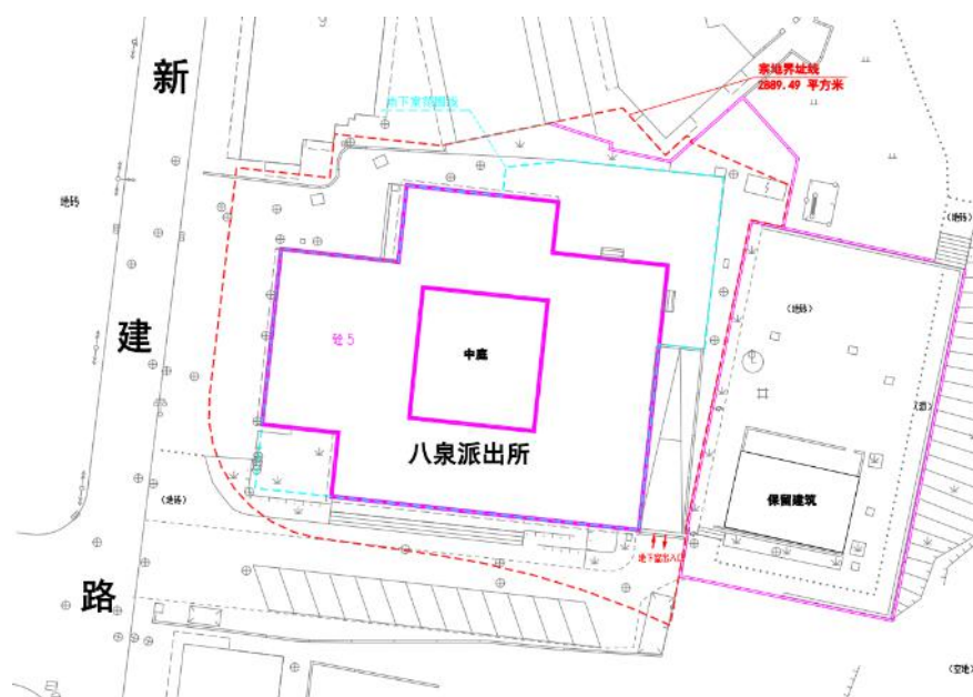
图二：竣工总平面图
