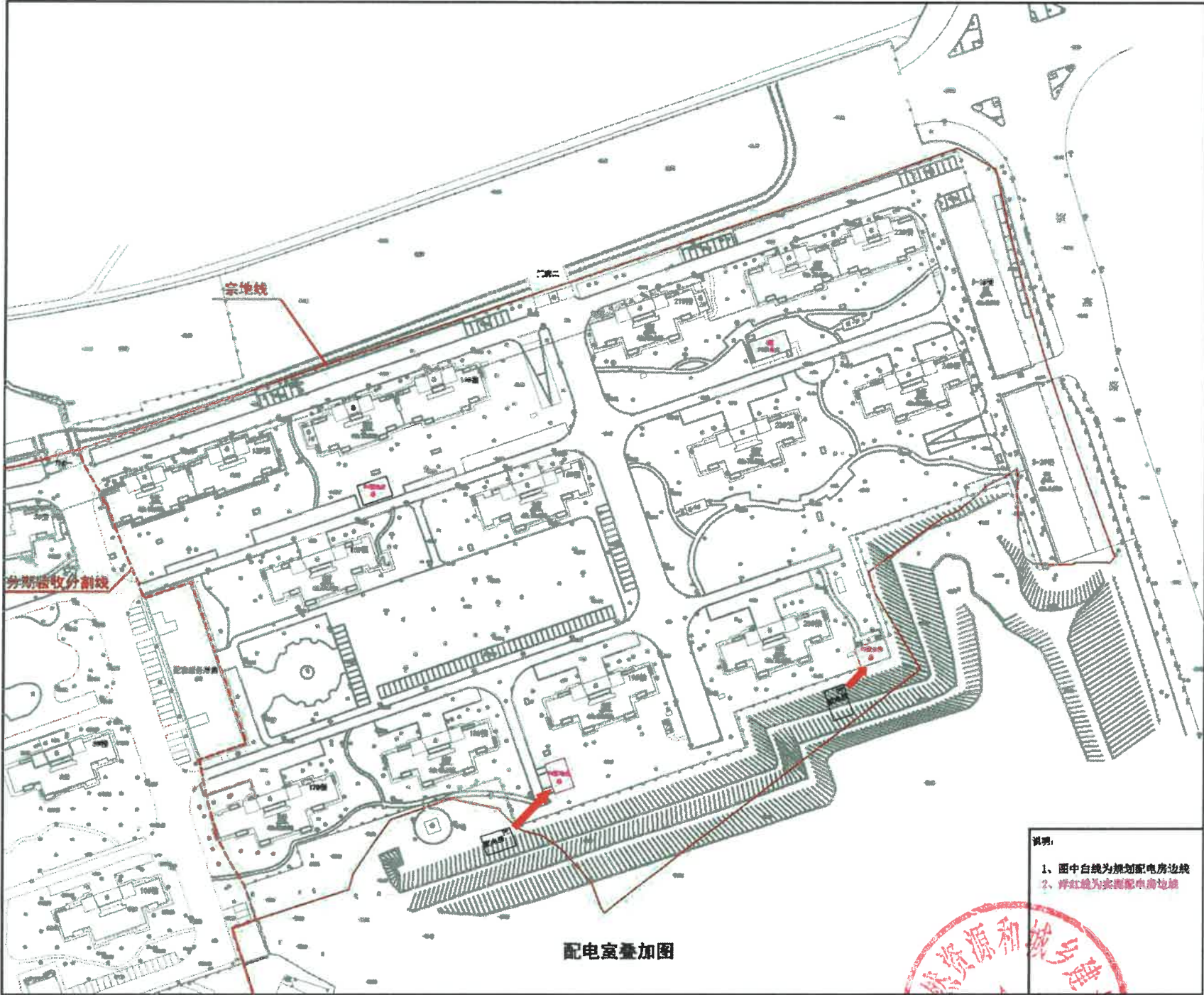
p5 配电房和 p7 配电房位置变更图
