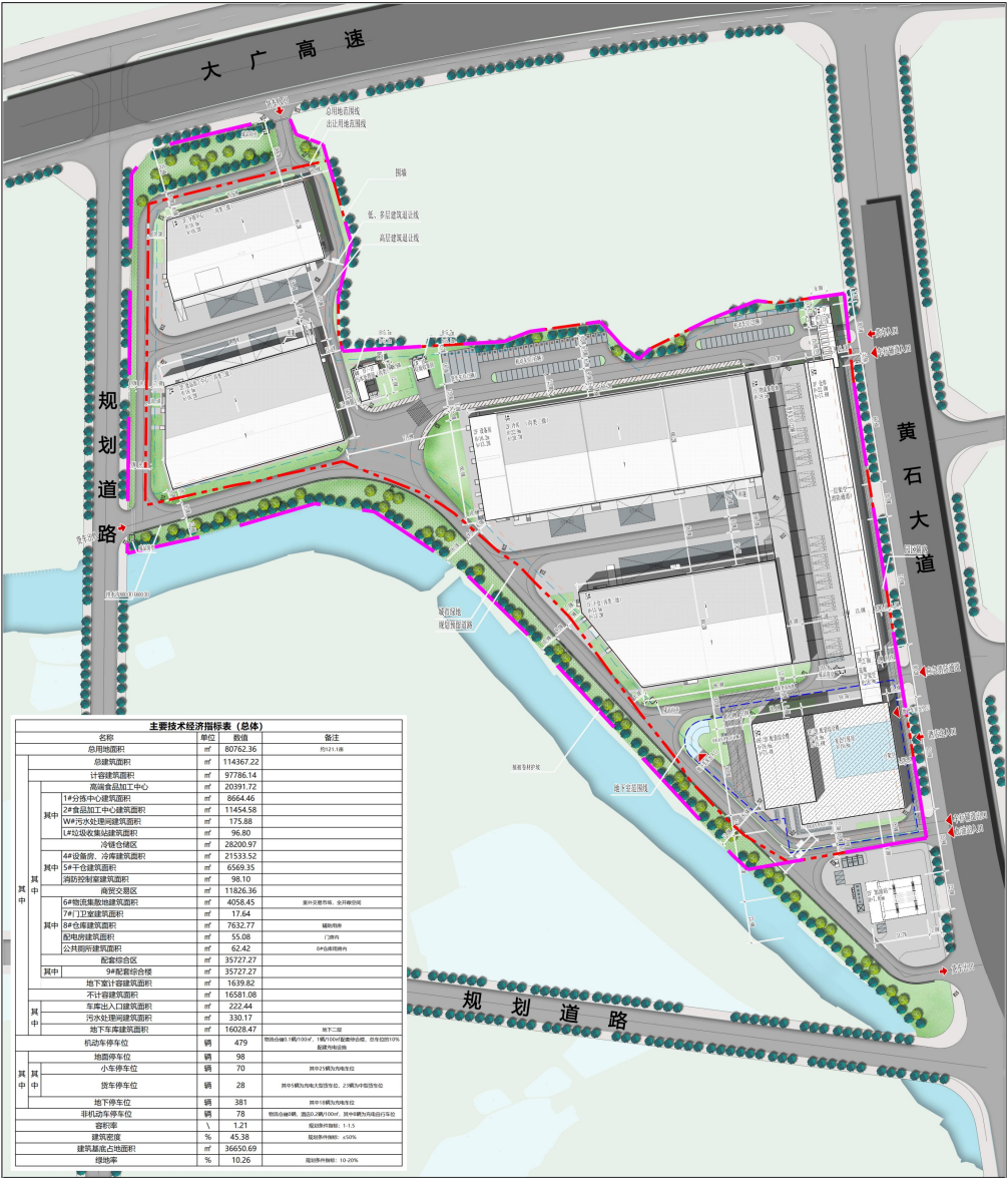
规划总平面图
