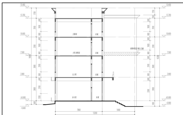
市级营房加建后剖面图
