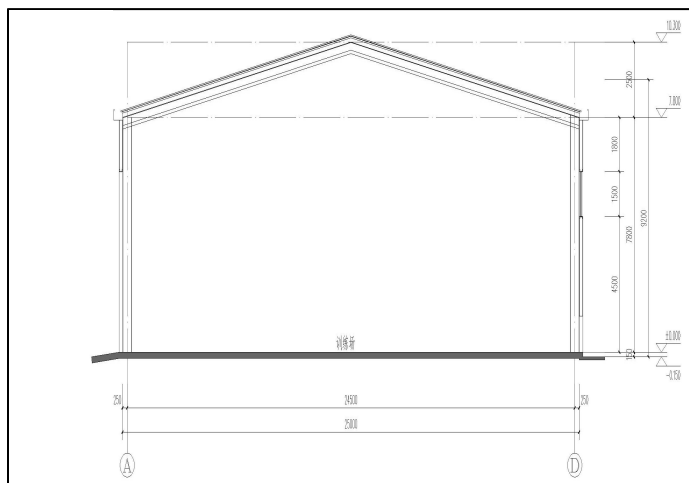
训练场剖面图
