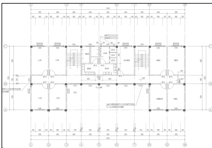
市级营房加建后三层平面图
