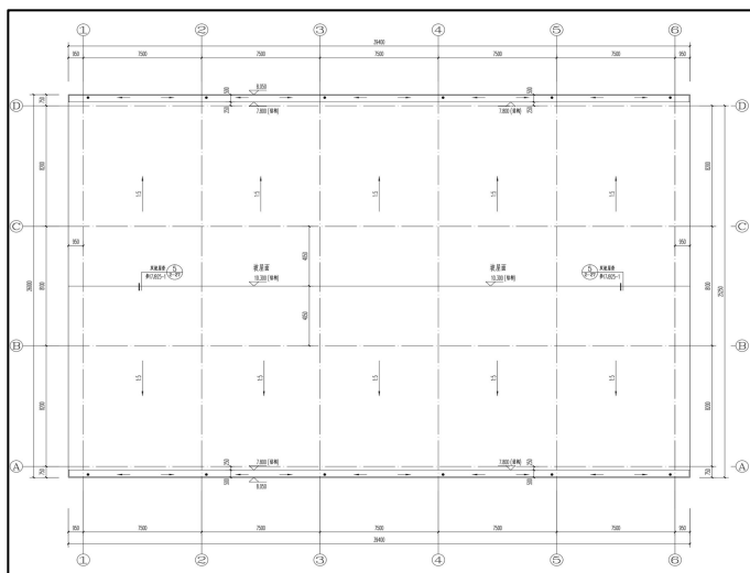
训练场屋顶层平面图
