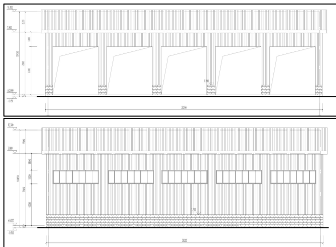
训练场立面图
