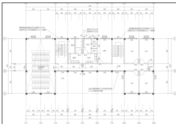
市级营房加建后四层平面图
