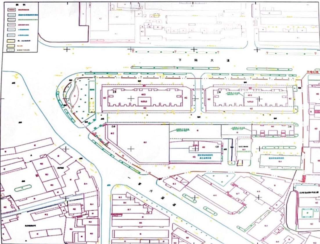
竣工总平面图
