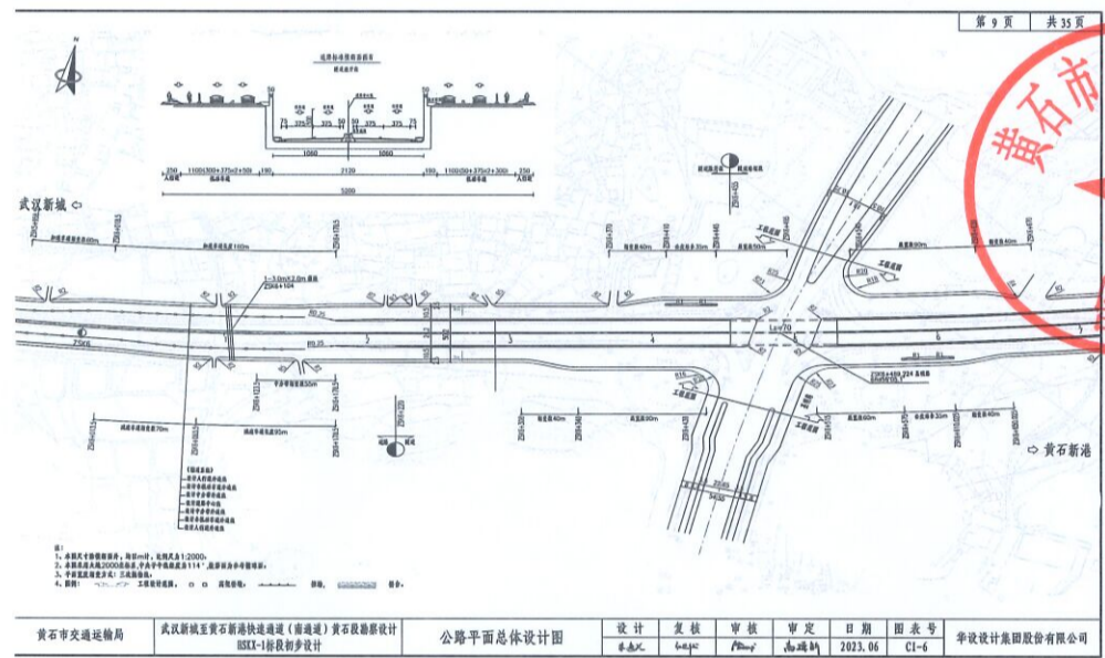
百花路交叉口平面图
