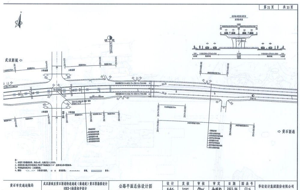
黄阳公路交叉口平面图
