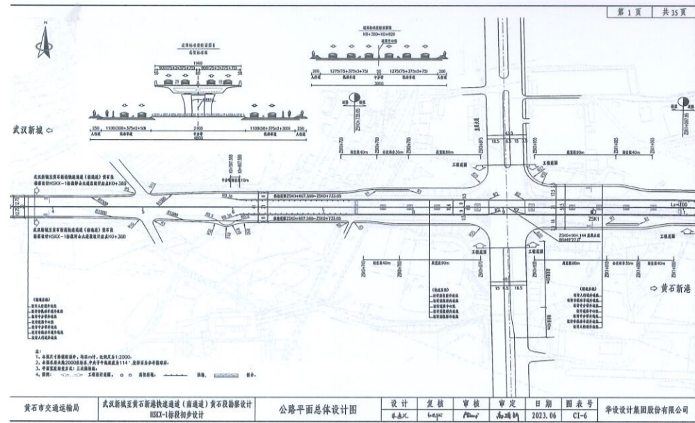
圣明路交叉口平面图
