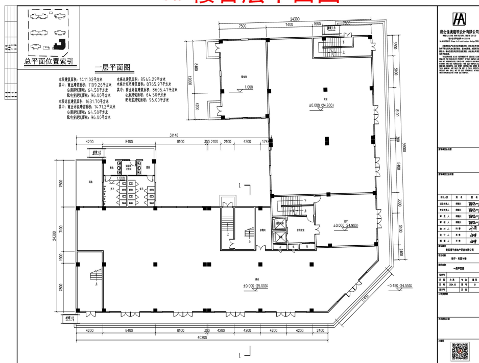
1# 楼三层平面图
