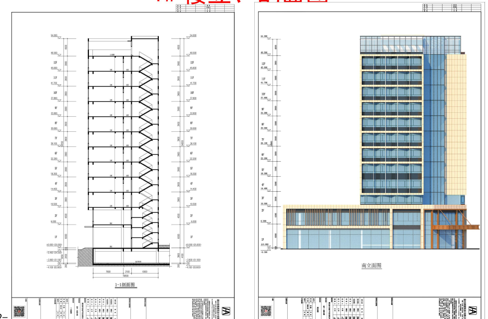
1# 楼立、剖面图
