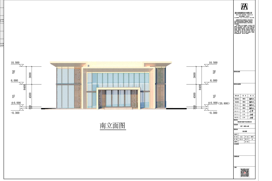
10# 楼建筑平、立、剖面图
