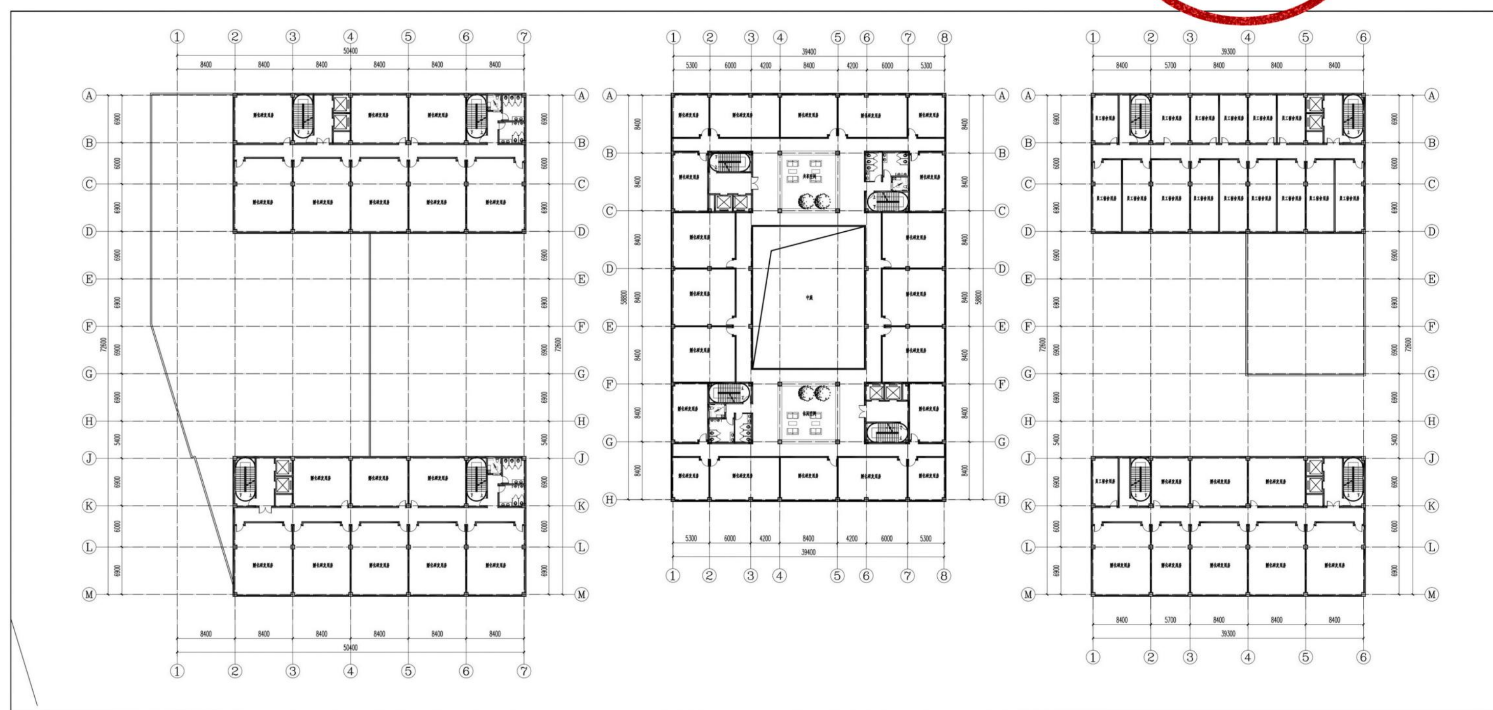
科创中心 4F 平面图
