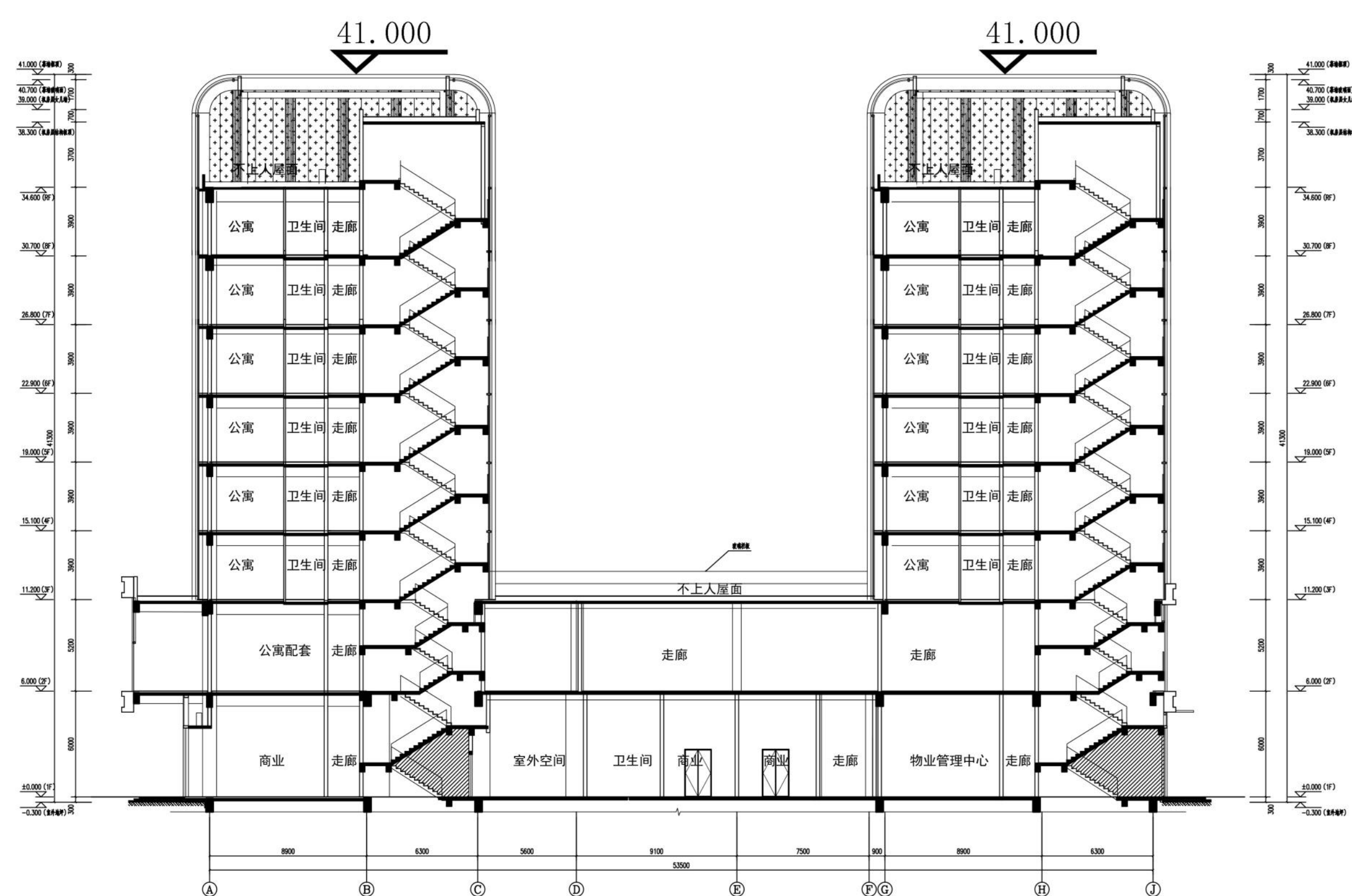
人才公寓剖面图
