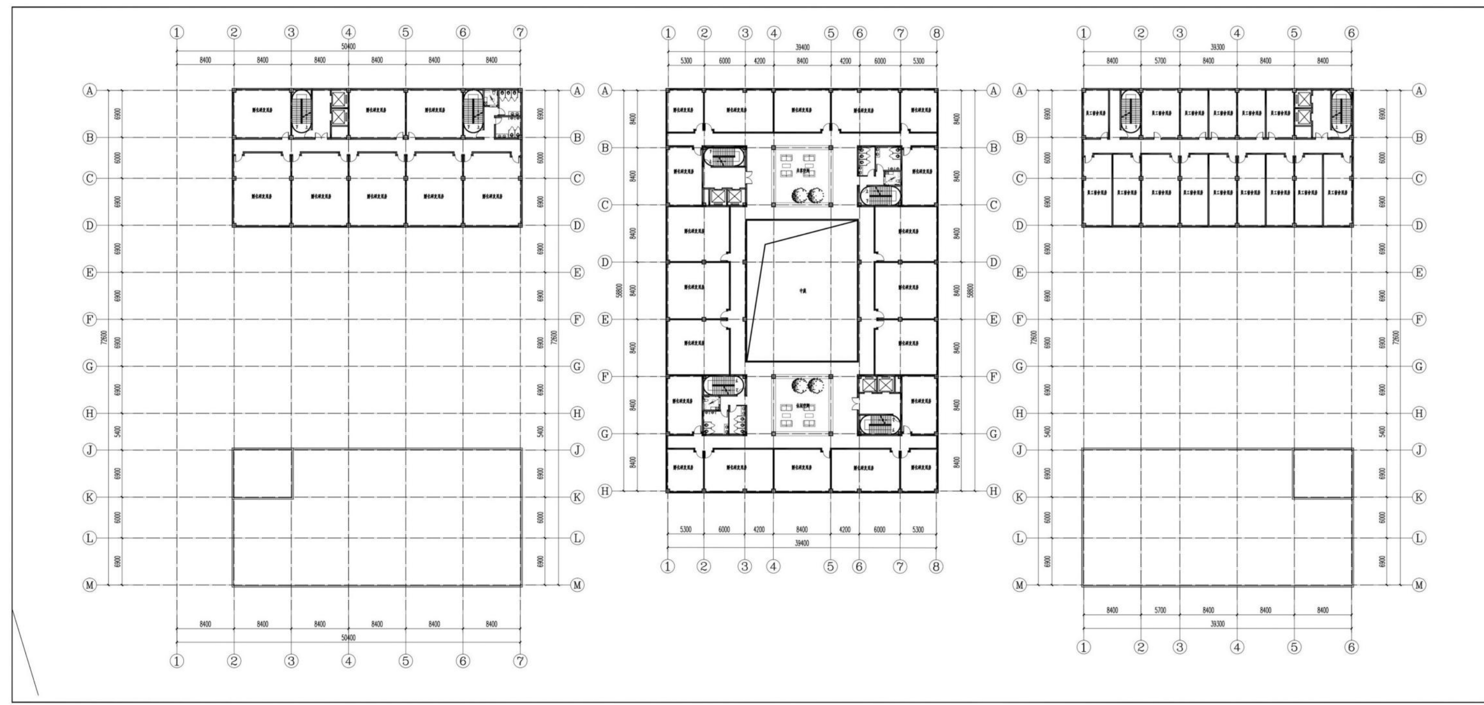
科创中心标准层平面图
