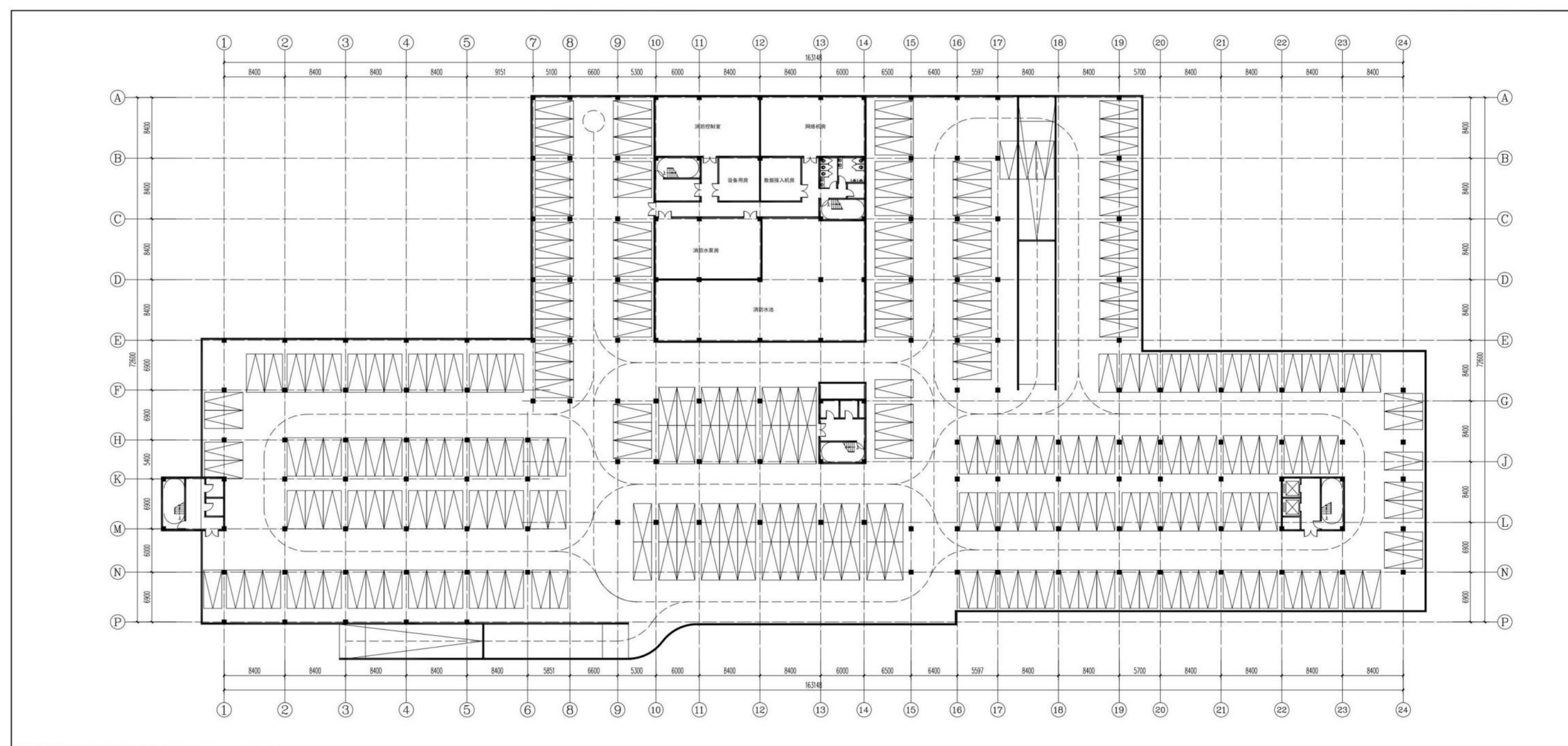
科创中心地下室平面图
