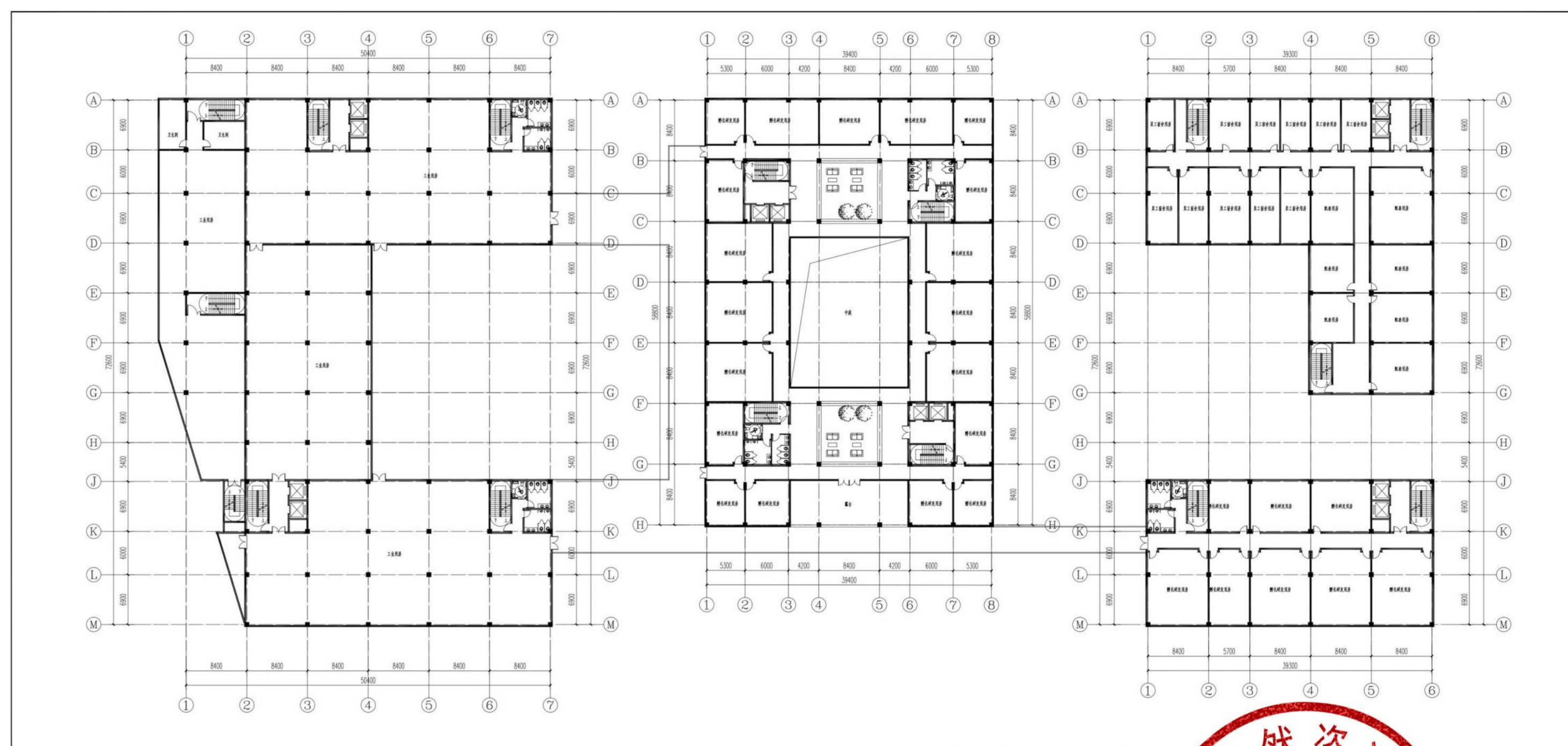
科创中心 2F 平面图
