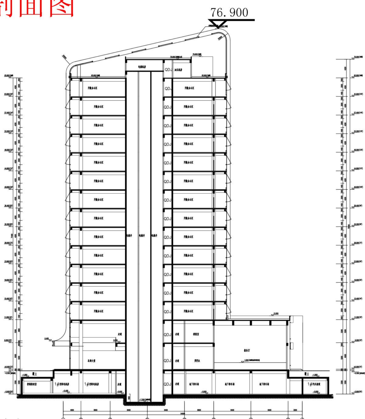
办公楼剖面图
