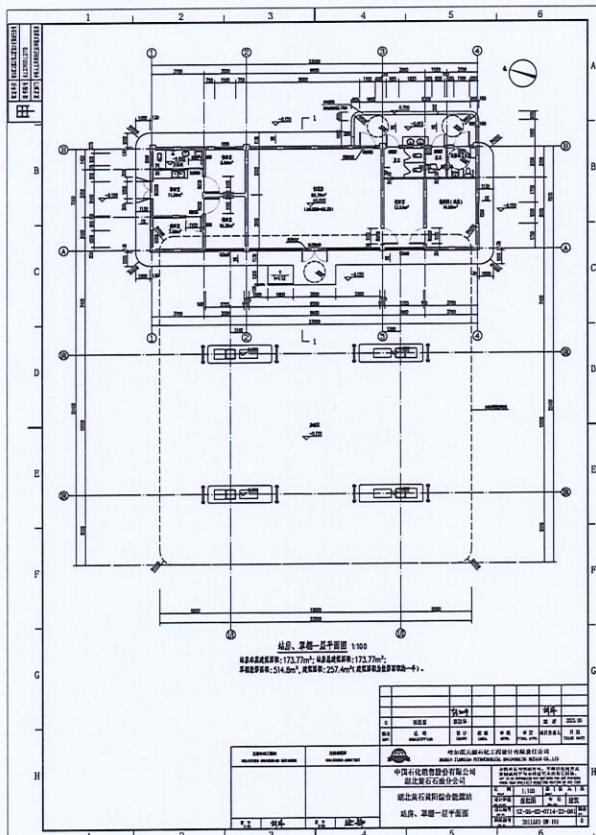
站房、罩棚一层平面图
