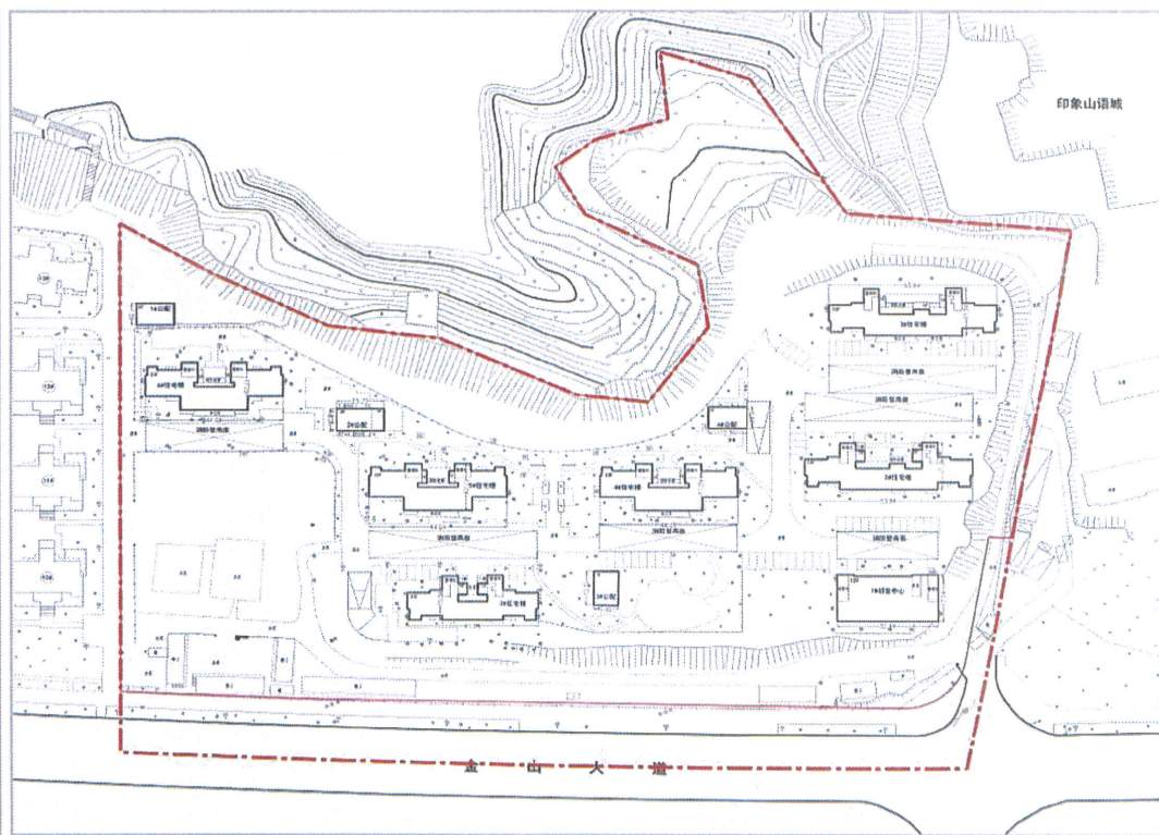
竣工总平面图
