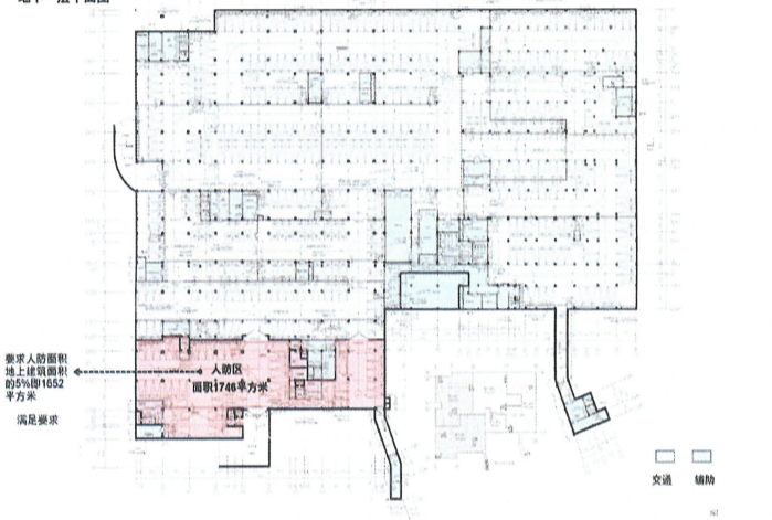
地下一层平面图
