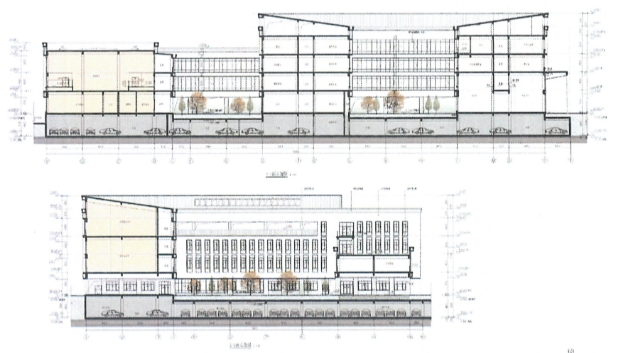
剖面图
