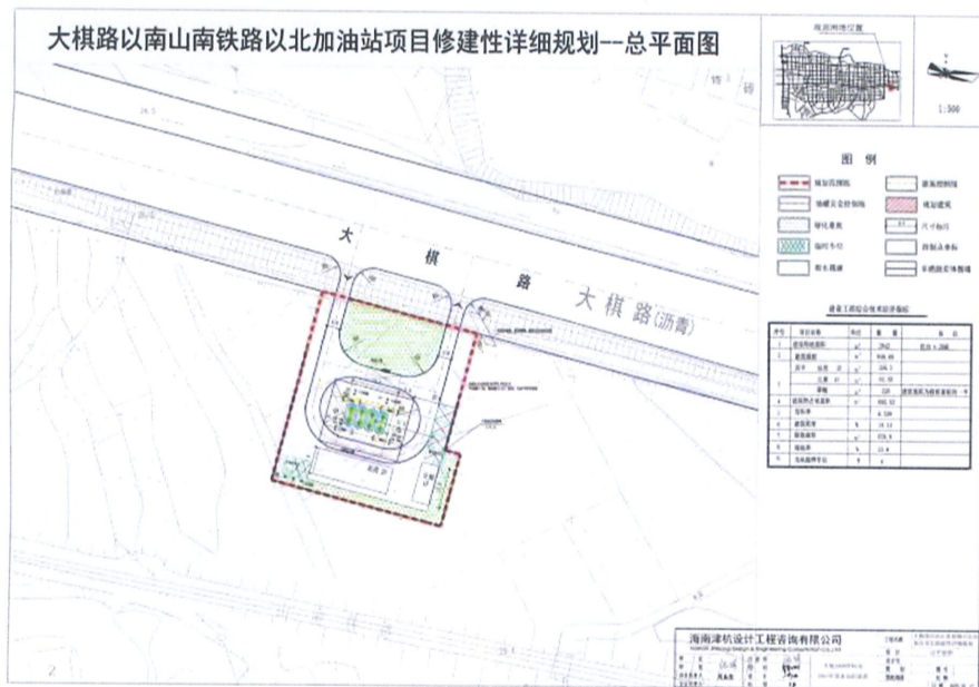
规划总平面图
