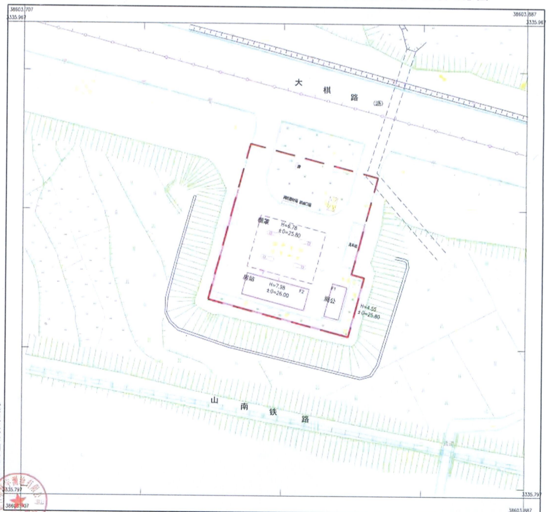
中国石油天然气股份有限公司湖北黄石月亮湾加油站竣工验收地形图
